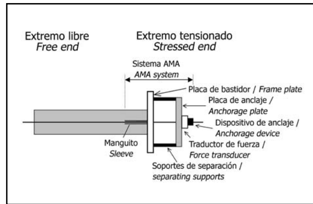
Figura 3. Esquema del sistema AMA. Figure 3. AMA system.
