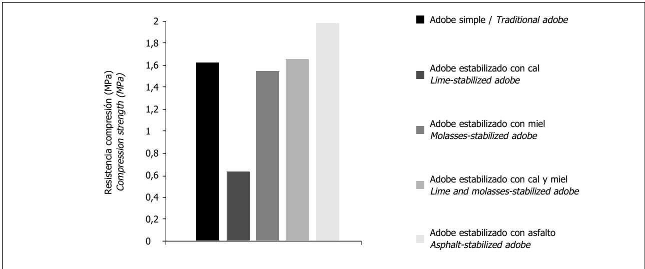
Figura 1. Comparación de los resultados del ensayo de compresión Figure 1. Comparison of compressive test results
