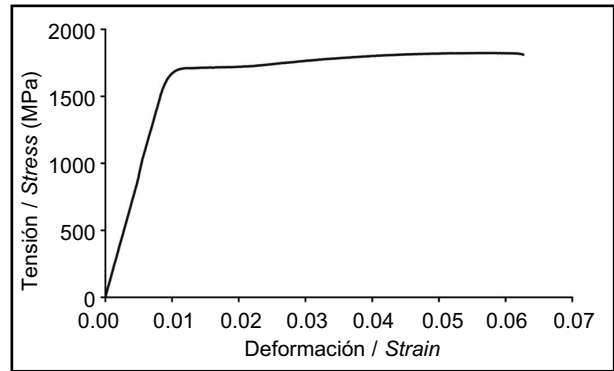
Figura 3. Curva tensión-deformación del alambre empleado en los ensayos.
