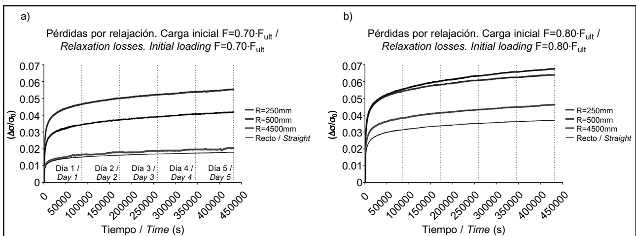
Figura 5. Evolución de las pérdidas por relajación en un ensayo a 120 h para cada uno de los radios de enrollamiento considerados: a) ensayos al 70% de la carga de rotura, b) ensayos al 80% de la carga de rotura. Figure 5. Development of relaxation losses in a 120 h relaxation test for each of the coiling diameters considered: a) tests at 70% of the ultimate tensile strength, b) tests at 80% of the ultimate tensile strength.
