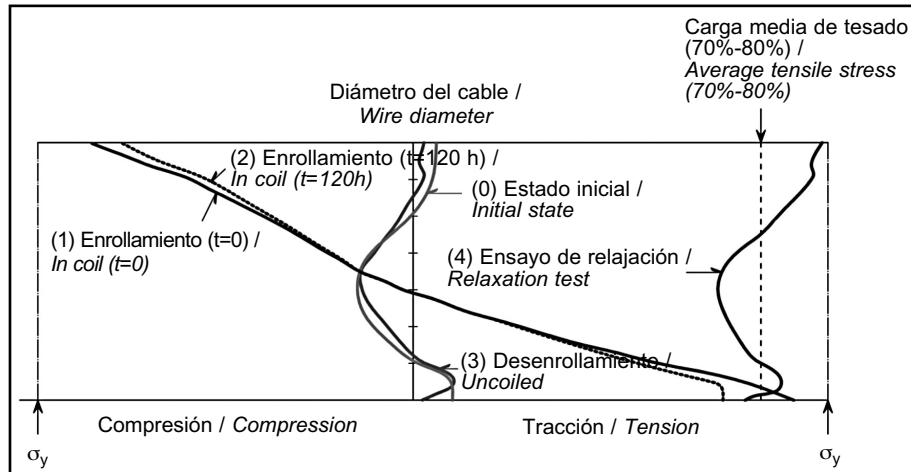
Figura 8. Perfiles de tensiones en la sección transversal de un cable con tensiones residuales durante el proceso de enrollamiento-desenrollamiento: (0) antes del enrollamiento, (1) recién enrollado, (2) tras 120 h enrollado, (3) una vez desenrollado, (4) una vez aplicada la carga del ensayo de relajación.
