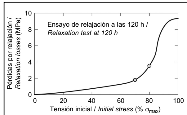
Figura 7. Comportamiento del alambre en un ensayo de relajación frente a diferentes cargas iniciales. Figure 7. Behaviour of a wire tested in a relaxation test under different initial loads.
