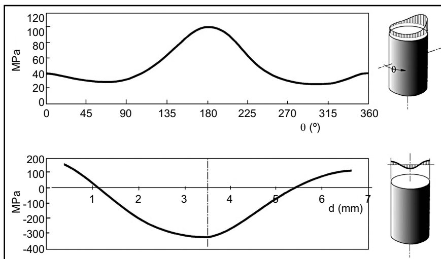
Figura 4. Tensiones residuales medidas en el alambre empleado en los ensayos: a) en el perímetro, b) a lo largo de un diámetro. Figure 4. Residual stresses measured on the tested wire: a) around the perimeter, b) along a diameter.
