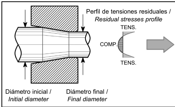
Figura 2. Esquema del proceso de trefilado y de las tensiones residuales generadas.
