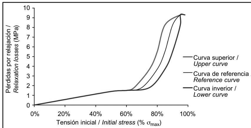
Figura 9. Curvas de relajación empleadas en el estudio de sensibilidad de esta curva sobre la relajación final. Figure 9. Relaxation diagrams used in sensitivity study of the curve on the final relaxation losses.
