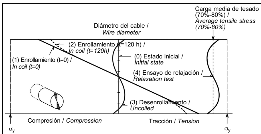
Figura 6. Perfiles de tensiones en la sección transversal de un cable sin tensiones residuales durante el proceso de enrollamiento-desenrollamiento: (0) antes del enrollamiento, (1) recién enrollado, (2) tras 120 h enrollado, (3) una vez desenrollado, (4) una vez aplicada la carga del ensayo de relajación.
