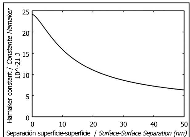
Figura 11. Constante efectiva de Hamaker en función de la separación entre partículas para la escoria sinterizada utilizando el software Hamaker (18). Figure 11. Effective Hamaker constant as a function of particle surface separation for sintered blast furnace slag using the Hamaker software (18).
