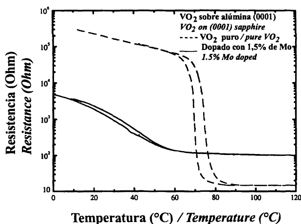
Figura 5.- Efecto del dopado con Mo sobre la temperatura de transición de fase de películas de \text{VO}_2 . Espesor de la película: 250 nm.
