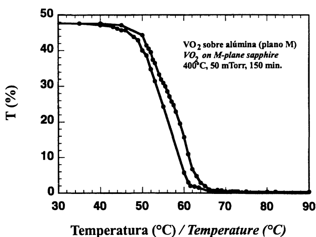
Figura 4.- Transmisión en el IR de películas de VO_2 bajo un ciclo térmico en el intervalo de 30 °C - 90 °C. Espesor de la película: 750 nm.
