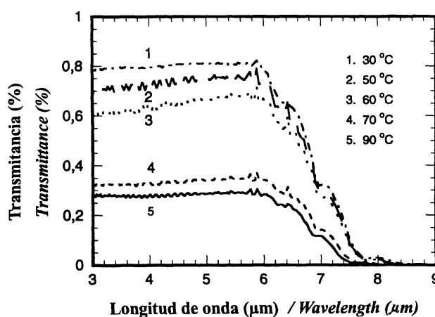
Figura 2.- Espectro de IR de películas de \text{VO}_2 bajo calentamiento. Espesor de la película: 100 nm
