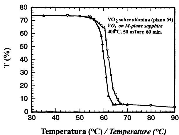
Figura 3.- Transmisión en el IR de la variación de la temperatura de tratamiento de películas de VO_2 desde 30 °C - 90 °C. Espesor de la película: 250 nm.
