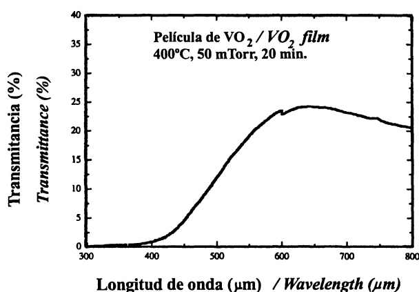
Figura 1.- Espectro UV de películas de \text{VO}_2 sobre zafiro según el plano M. Espesor de la película: 100 nm.
