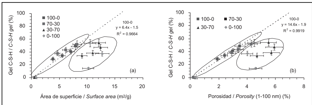
Figura 3. Correlaciones cuantitativas obtenidas entre el gel C-S-H, (a) área superficial y (b) porosidad de 1-100 nm de diámetro. Figure 3. Quantitative correlations obtained among the C-S-H gel, (a) surface area and (b) porosity of 1-100 nm of diameter.
